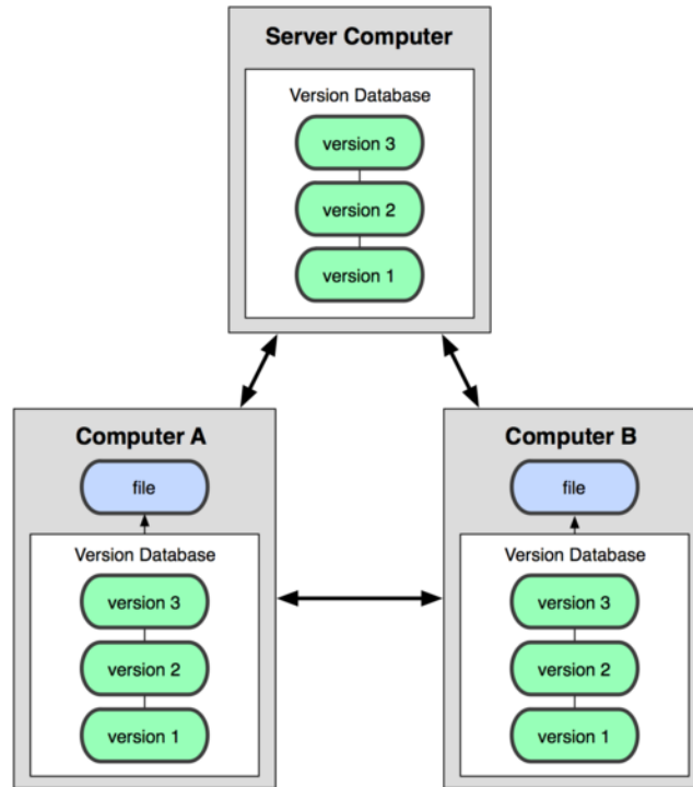
그림 1.3: 분산형 버전 관리 시스템(DVCS) 다이어그램.
