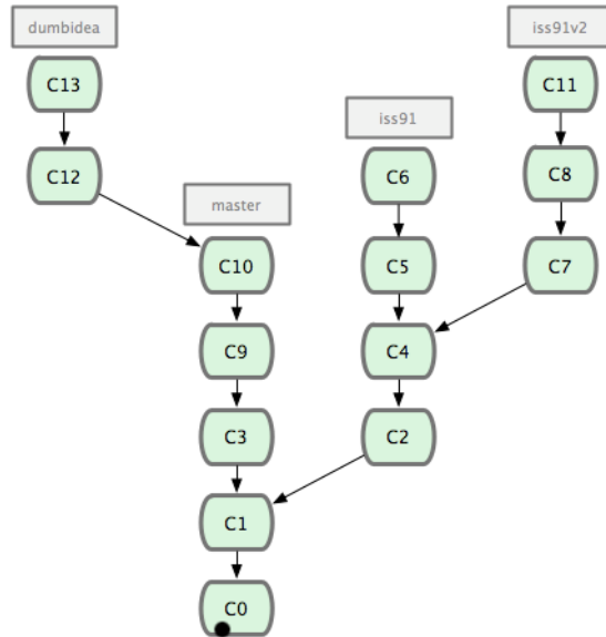
그림 3.20: 여러 토픽 브랜치에 대한 커밋 히스토리
