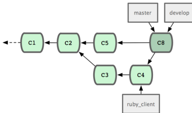
그림 5.23: 토픽 브랜치를 Release한 후.
