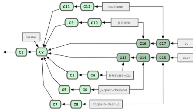
그림 5.25: 토픽 브랜치를 긴 호흡의 통합 브랜치로 Merge하기.
