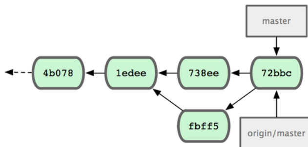
그림 5.6: Push하고 난 후, John씨의 저장소.
