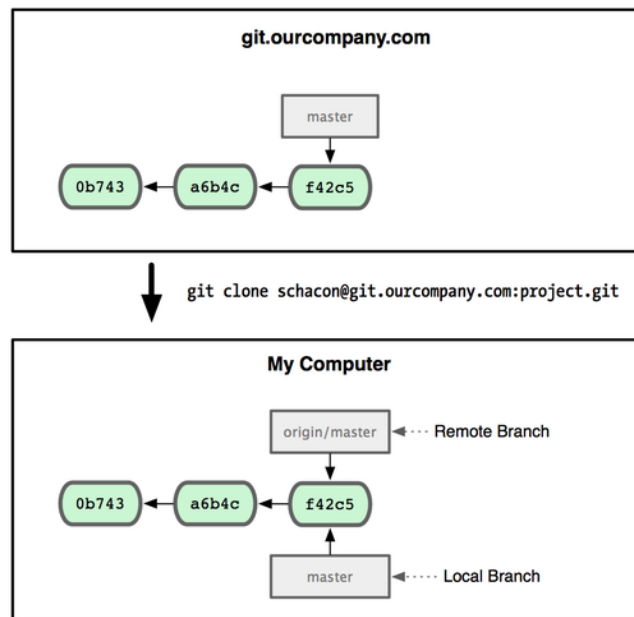
그림 3.22: 저장소를 Clone하면 로컬 master 브랜치, 리모트 저장소의 master 브랜치를 가리키는 origin/master 브랜치가 생긴
