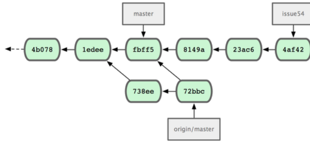
그림 5.8: John씨의 커밋을 Fetch한 후 Jessica씨의 저장소.
