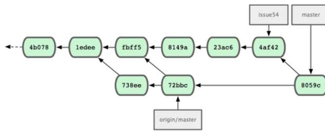
그림 5.9: Merge 이후 Jessica씨의 저장소.
