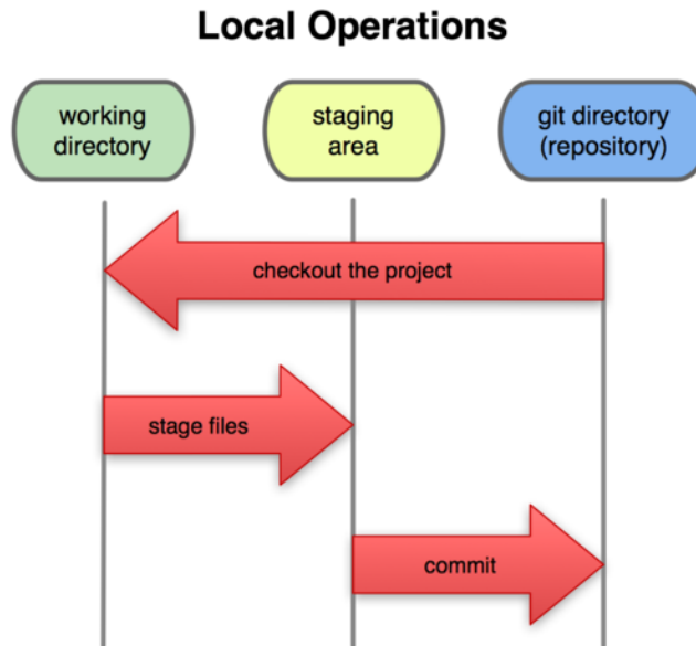
그림 1.6: Working Directory, Staging Area, Git Directory
