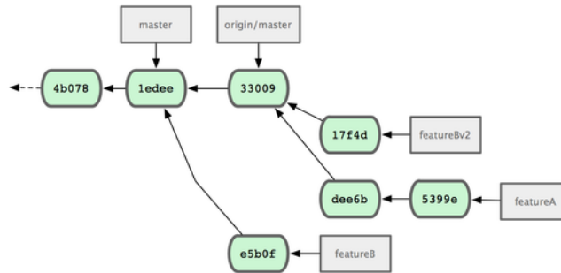
그림 5.18: featureBv2 브랜치를 Commit한 이후 저장소의 모습.
