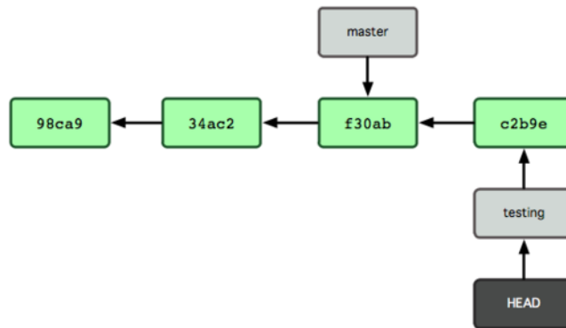
그림 3.7: HEAD가 새 커밋을 가리키는 testing 브랜치의 모습
