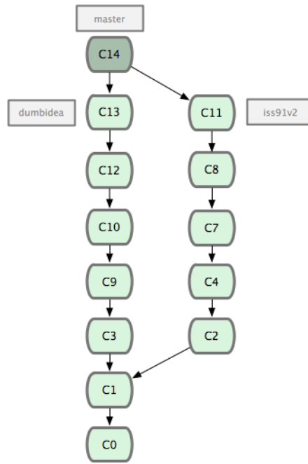
그림 3.21: dumbidea와 iss91v2 브랜치를 Merge하고 난 후의 모습
