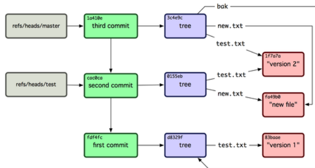
그림 9.4: 브랜치 레퍼런스가 추가된 Git 데이터베이스
