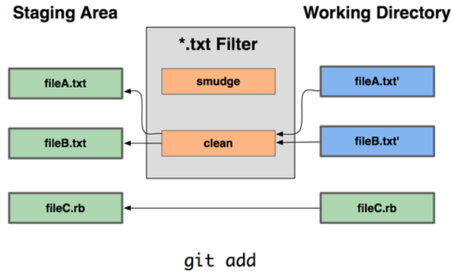
그림 7.3: “clean” 필터는 파일을 Stage할 때 실행된다.
