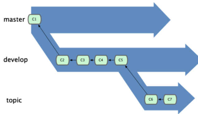
그림 3.19: 각 브랜치를 하나의 실험실로 생각하면 쉽다.
