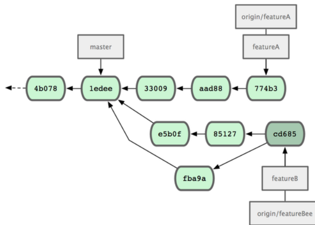
그림 5.13: 마지막 Push하고 난 후의 Jessica씨의 저장소
