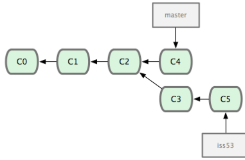
그림 3.15: master와 별개로 진행되는 iss53 브랜치
