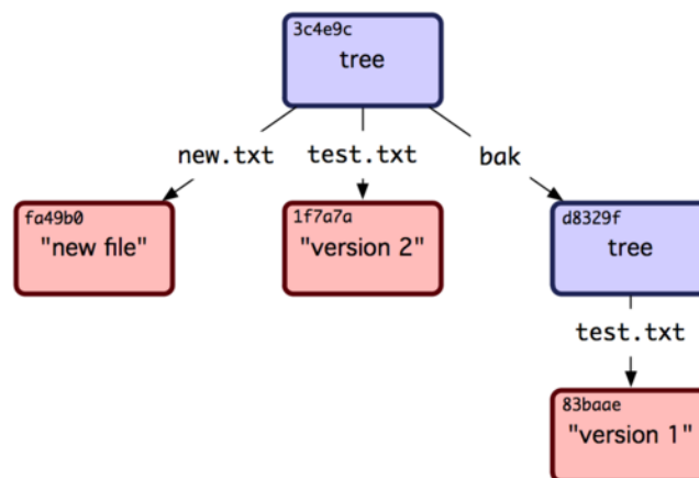
그림 9.2: Git 데이터 구조.
